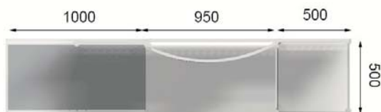
TOP ELEVATION
